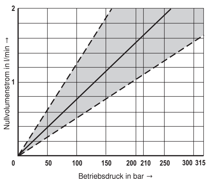
Typ 4WREE 10 V75
